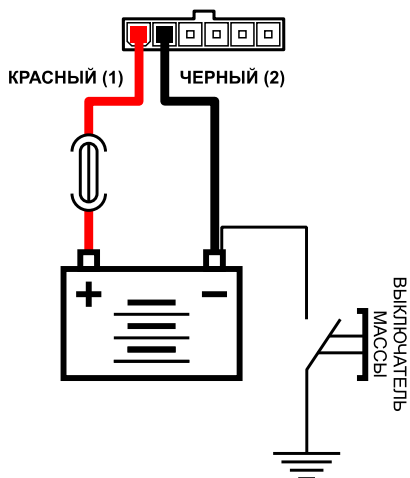
Подключение питания до выключателя массы
