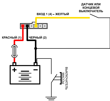
Схема до выключателя массы
