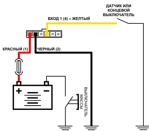
Схема после выключателя массы
