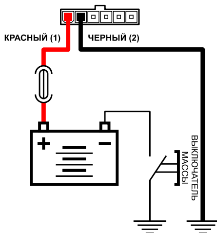
Подключение питания после выключателя массы
